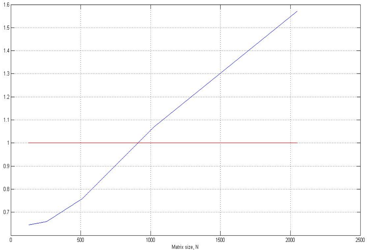
Рисунок 2 – Ускорение параллельного алгоритма
