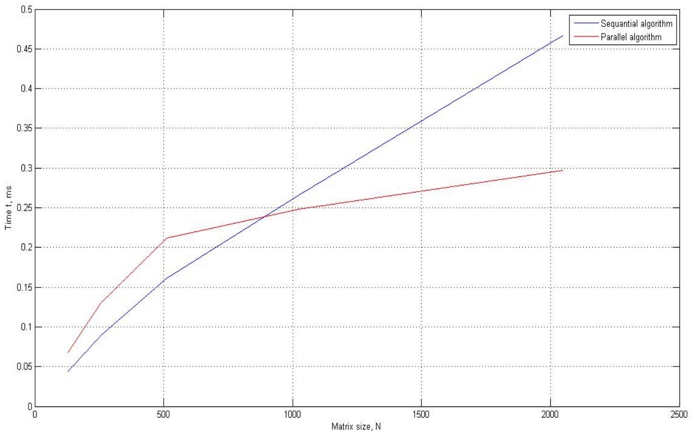
Рисунок 1 – Время работы алгоритмов
